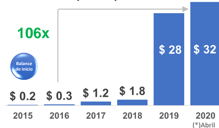
RATIOS FINANCIEROS
